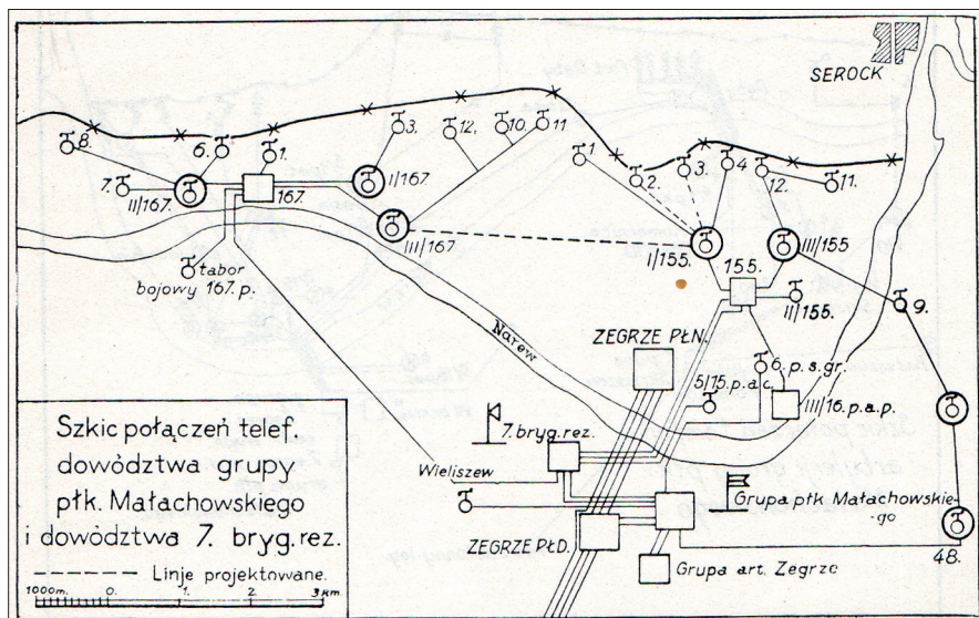
Schemat łączności odcinka „Zegrze”
