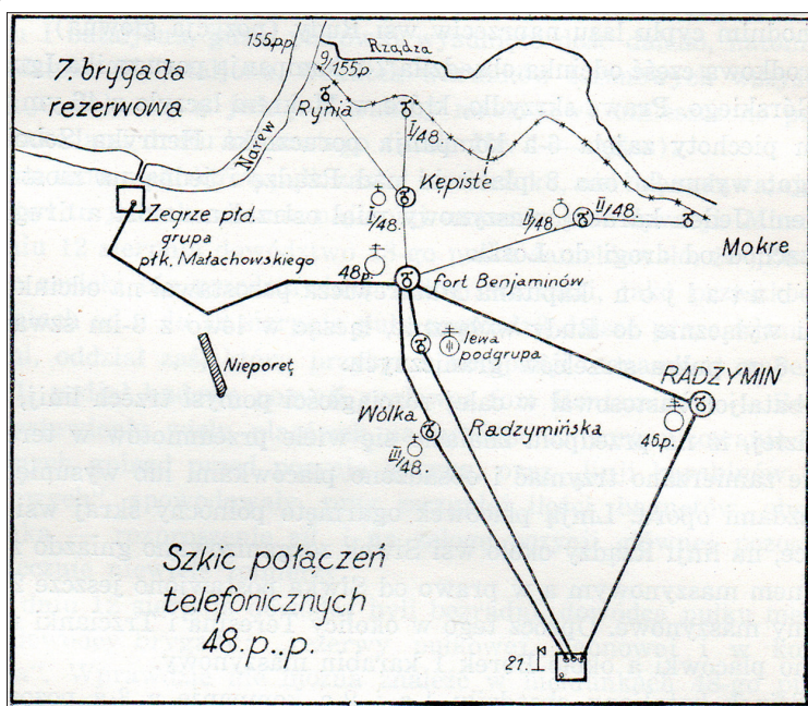
Schemat łączności 48. Pułku Piechoty (B. Waligóra, Bój na przedmościu Warszawy w sierpniu 1920 r. , Warszawa 1934, s. 83.)
