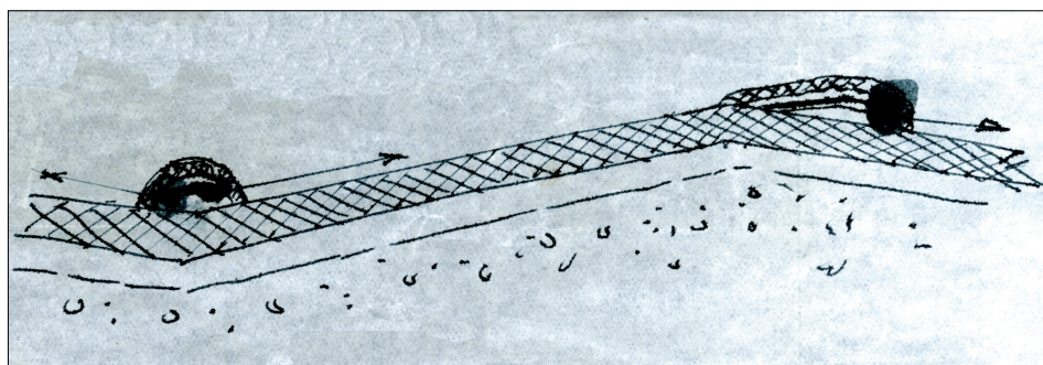
Rowy strzeleckie wraz z pozycjami flankującymi wg instrukcji wykonania robót fortyfikacyjnych na pododcinku „Zegrze” (CAW, Relacje i wspomnienia, sygn. I.400.1505.P, s. 95)
